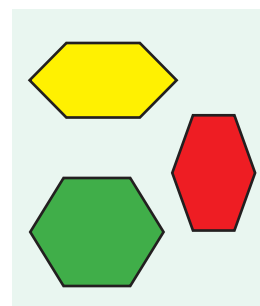
Шестикутники
