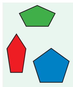
П'ятикутники
