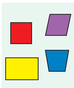
Чотирикутники
