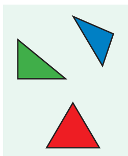
Трикутники
